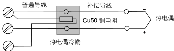
(2) 外接铜电阻自动补偿模式
