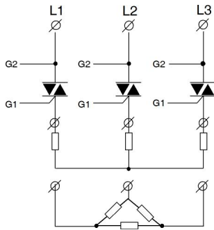
K3 三相三线星型、 三角型接线图（双向可控硅）
